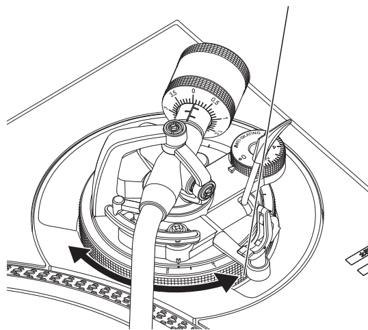
Ручка [HEIGHT ADJUST]
