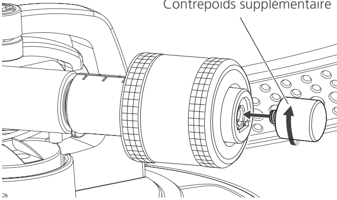
Contrepois supplémentaire
