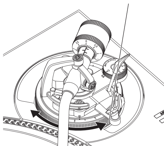
Botão rotativo [HEIGHT ADJUST]
