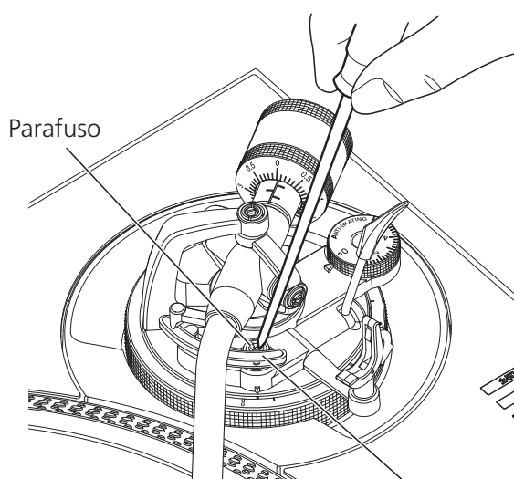
Elevador do braço
