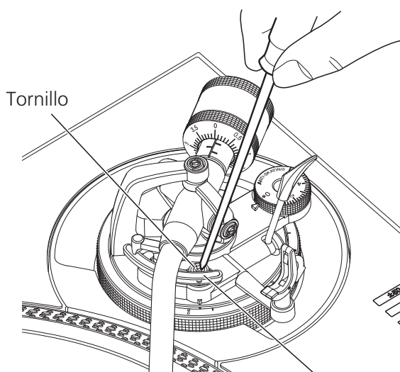
Elevador del brazo
