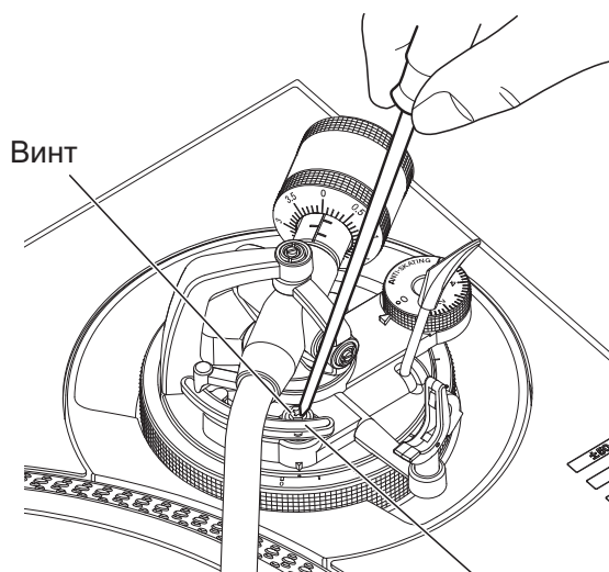
Микролифт тонарма
