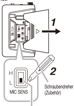
Mikrofonempfindlichkeits-Wählschalter
