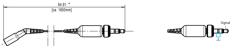
Kabel mit 3,5 mm Klinenstecker / cable with 3.5 mm jack plug
