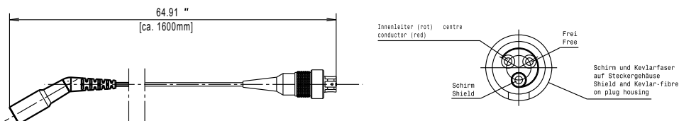
Kabel mit 3-poligem Spezialstecker / cable with 3-pin special connector
